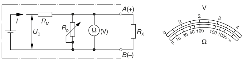
Bild 2.7 Parallelohmometer; U_B Betriebsspannung der Batterie; R_M Vorwiderstand; R_P veränderlicher Parallel- bzw. Nebenwiderstand; R_X Widerstand des Prüflings
