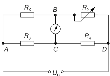
Bild 2.8 Wheatstone-Brücke
