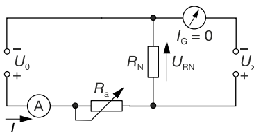
Bild 2.4 Lindeck-Rothe-Kompensator
